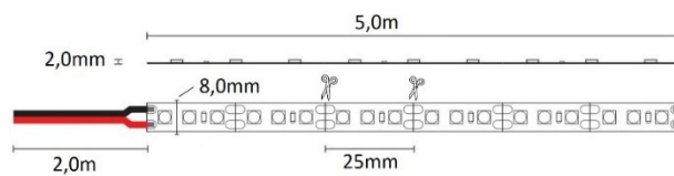
9,6W nauhan mitat ja katkaisukohdat
