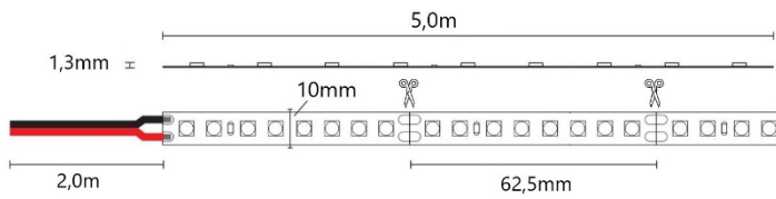
17,2W nauhan mitat ja katkaisukohtat
