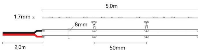
COB 10W 24V nauhan mitat ja katkaisukohtat
